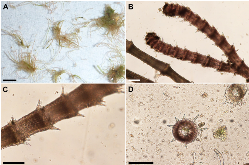
Figure 3 : Centrocercus clavulatum (Agardh) Montagne A. Les thalles de Centrocercus clavulatum récoltés à Bréhat en septembre 2017. B. Détail d'un thalle montrant la pseudo-dichotomie. C. Détail des cellules corticales rectangulaires. D. Coupe transversale d'un thalle montrant le verticille d'épines. Barres d'échelles : A : 1 cm ; B, C, D : 100 \mu m. (Photos : Michel Le Duff).
